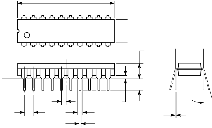
SCALE 1:1
